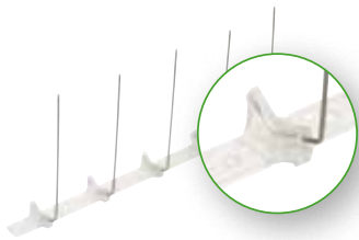
Hroty BIRDEX T1 dílek 25 cm (kat. č. 467001)
